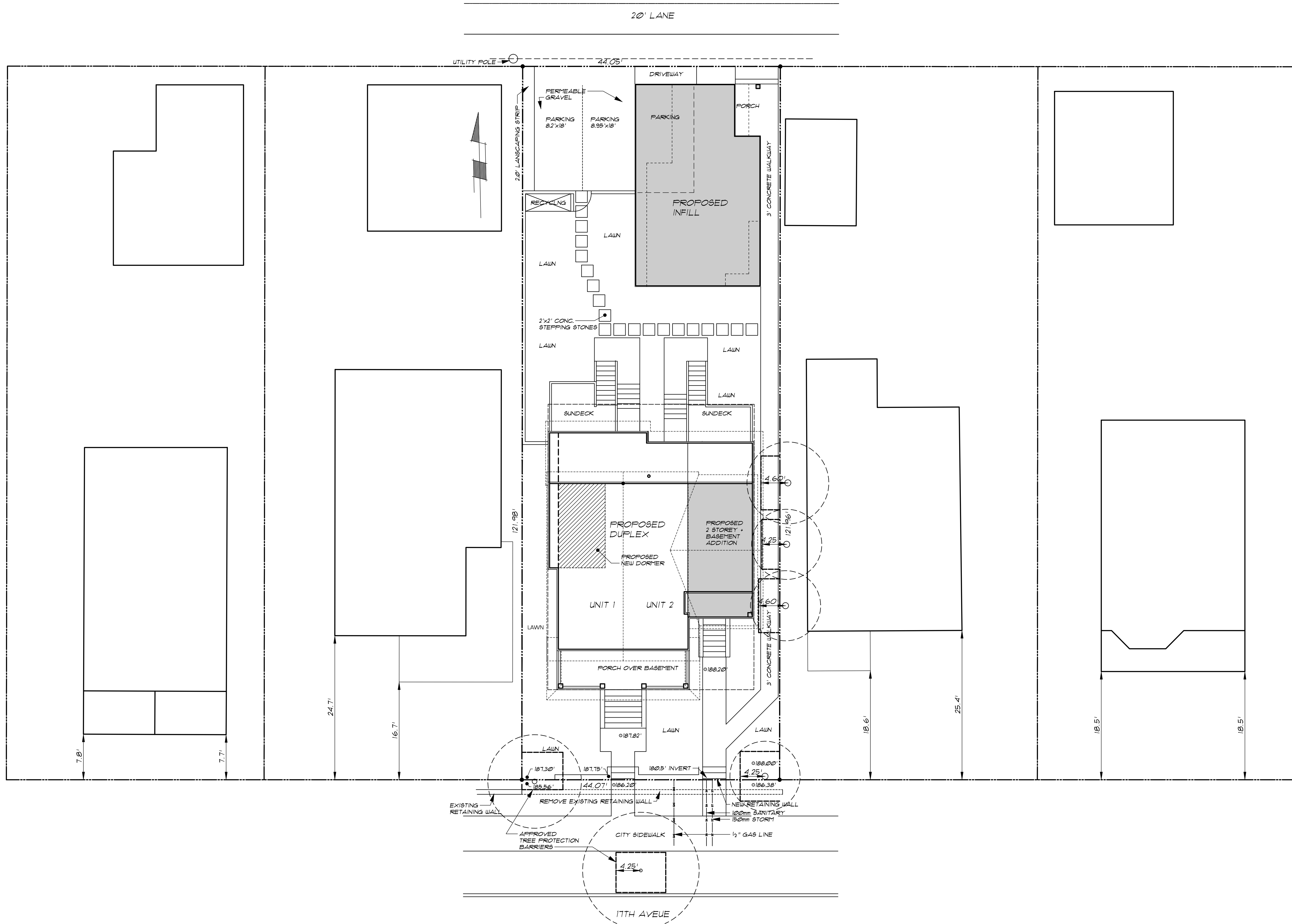
context plan scale: 1"=8'
