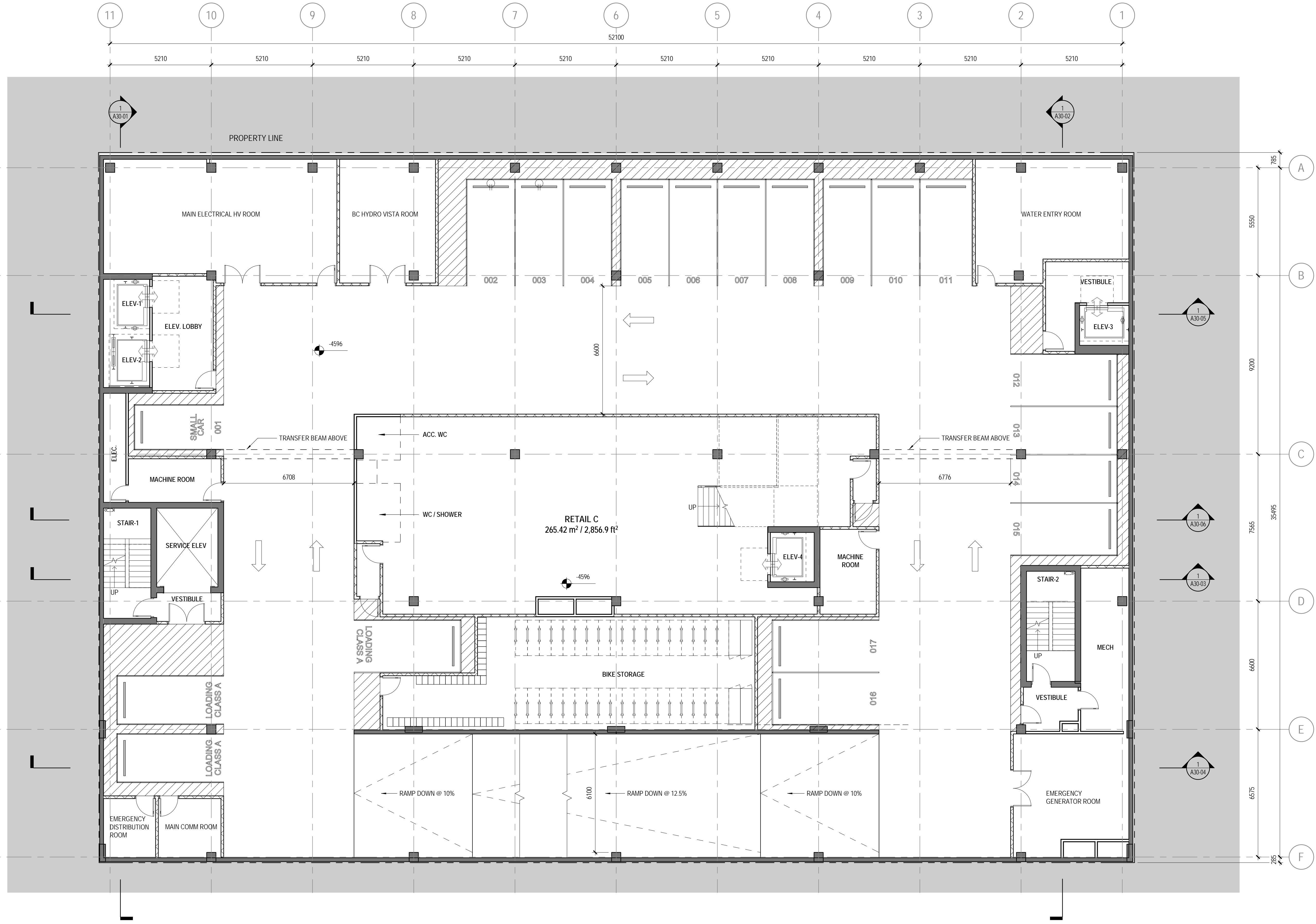
1 LEVEL P1 1 : 100
