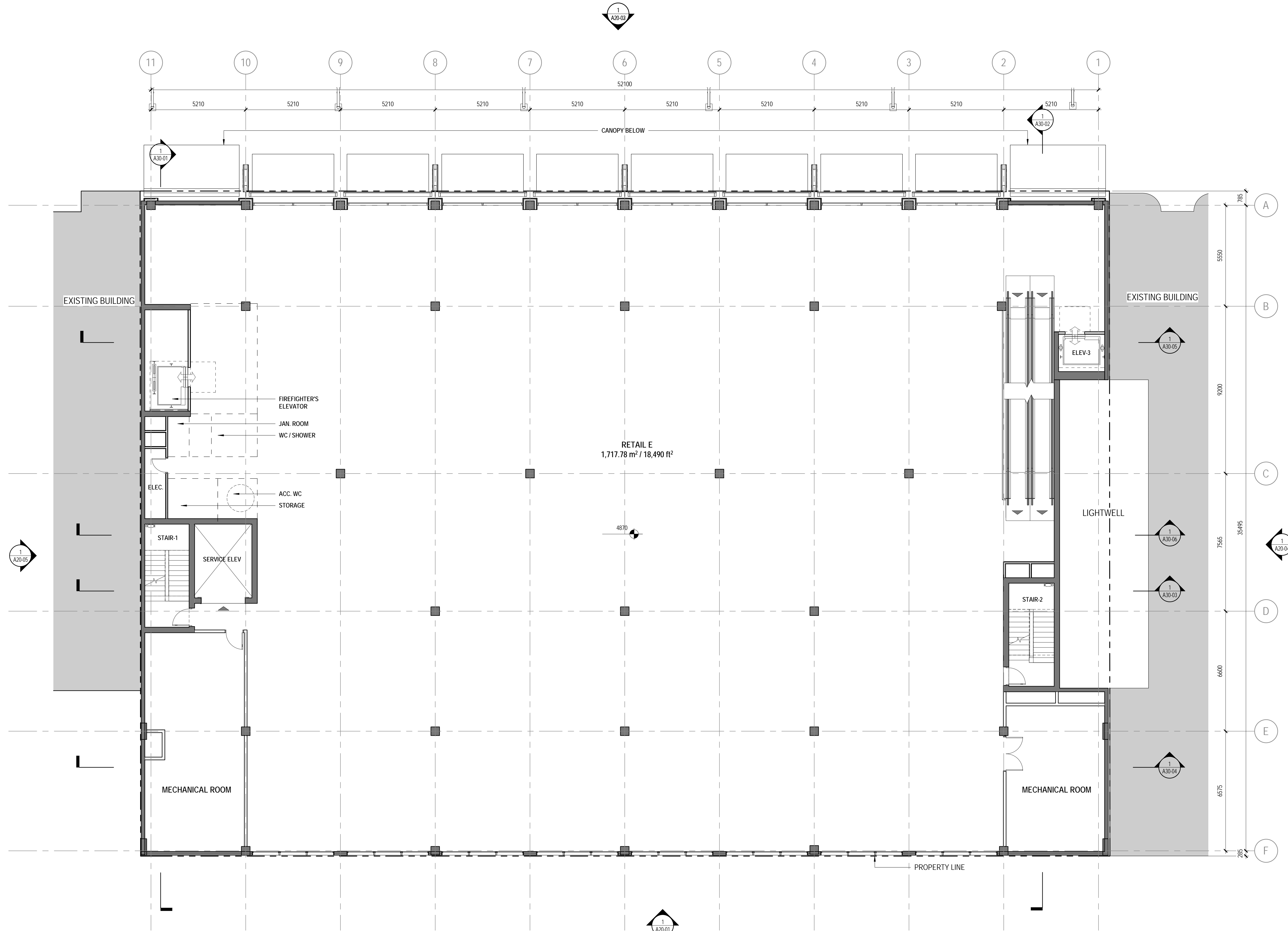
1 LEVEL 02 1 : 100
