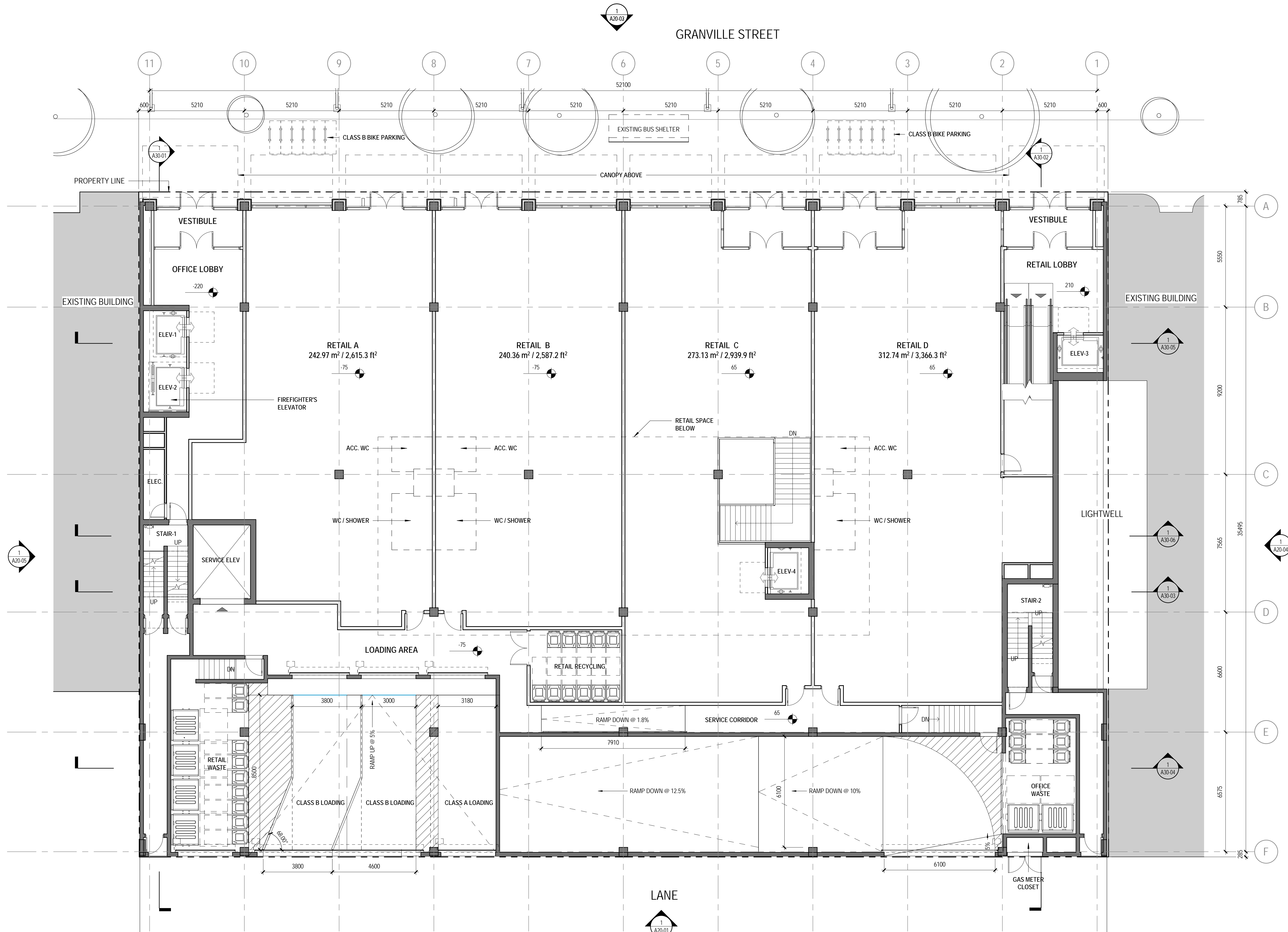
1 LEVEL 01 1 : 100
