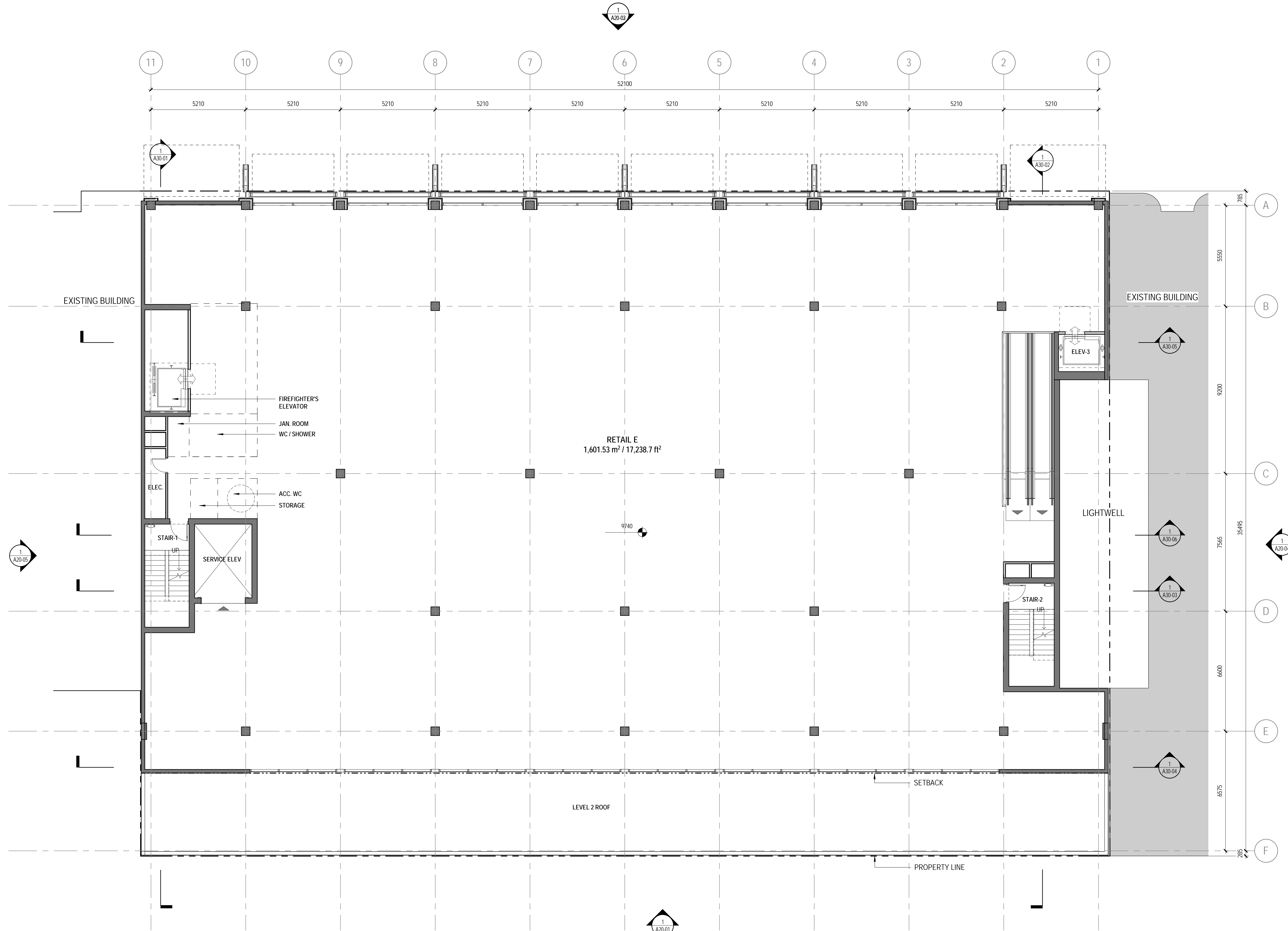
① LEVEL 03 1:100
